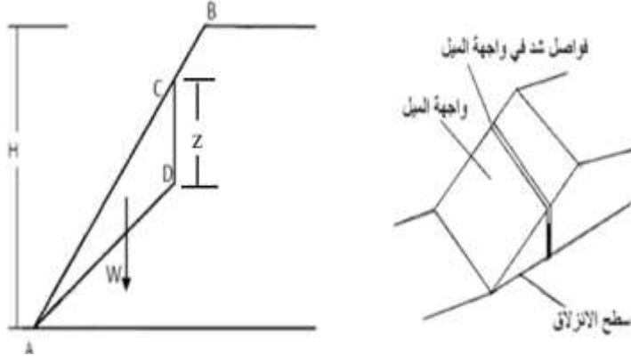
الشكل 6: كتلة صخرية في حالة وجود فواصل الشد في السطح المائل
