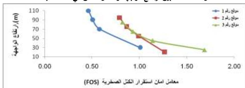
شكل 10: العلاقة بين ارتفاع الواجهة ومعامل الأمان في حالة التشبع الغير كامل
