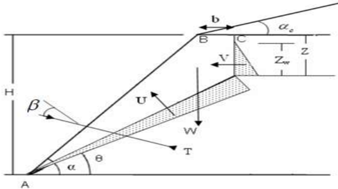
شكل 8: الانهيار المستوي مع فواصل في اعلي الميل مع وجود تثبيت بمسامير الصخر
