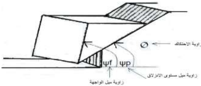
شكل 2: الانهيار المستوي
