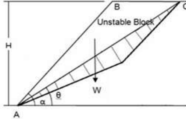
شكل 4 : انزلاق الكتلة الصخرية المشبعة بالمياه
