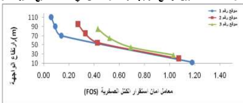
شكل 10: العلاقة بين ارتفاع الواجهة ومعامل الأمان في حالة التشبع الغير كامل
