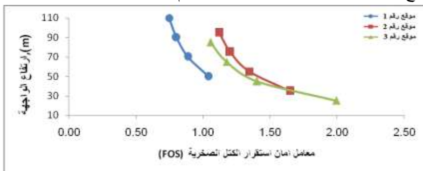
شكل 9: العلاقة بين ارتفاع الواجهة ومعامل الأمان في الحالة الجافة
