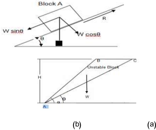
شكل 3 : مخطط ميل الانهيار المستوي
