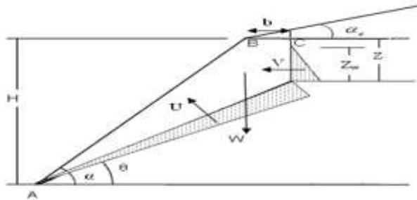
شكل 7: الانهيار المستوي مع وجود ميل وفواصل الشد تحت زاوية الميل
