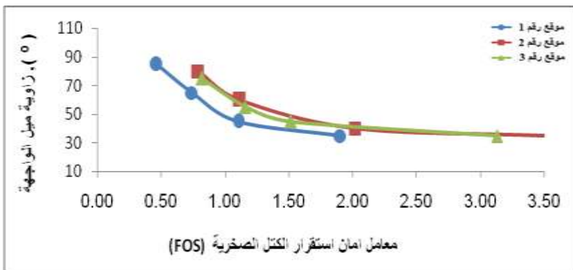
شكل 13: العلاقة بين زاوية ميل الواجهة ومعامل الأمان في حالة عدم التشبع الكامل
