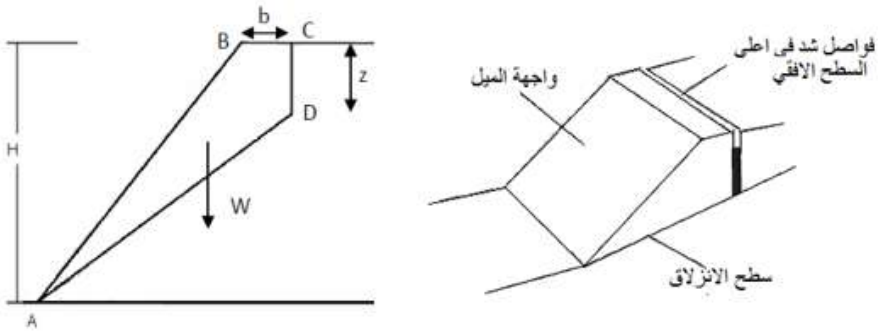
شكل 5 : كتلة صخرية في حالة وجود فواصل الشد في السطح المستوي العلوي
